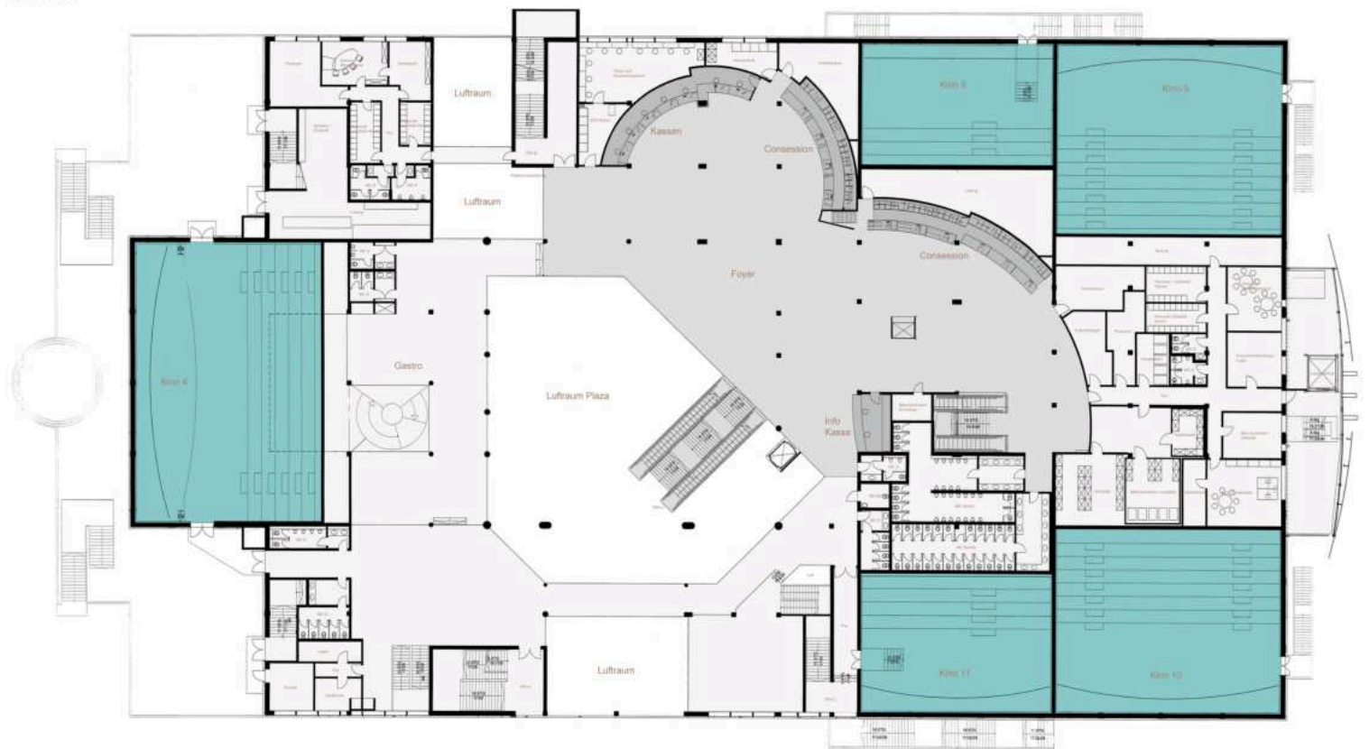
1.Obergeschoss M 1:100
