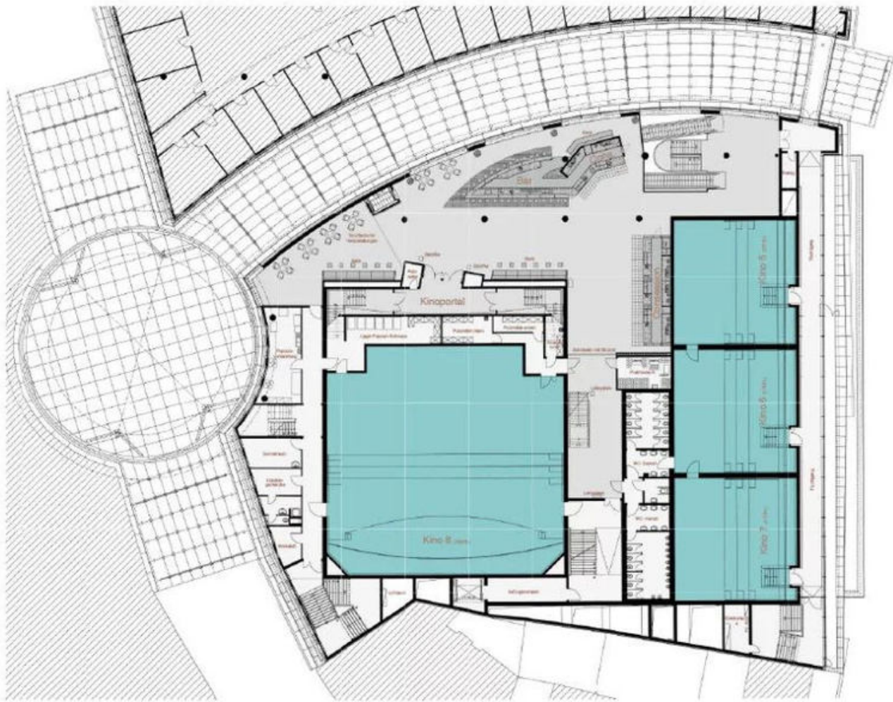
Grundriss: 4. OG
